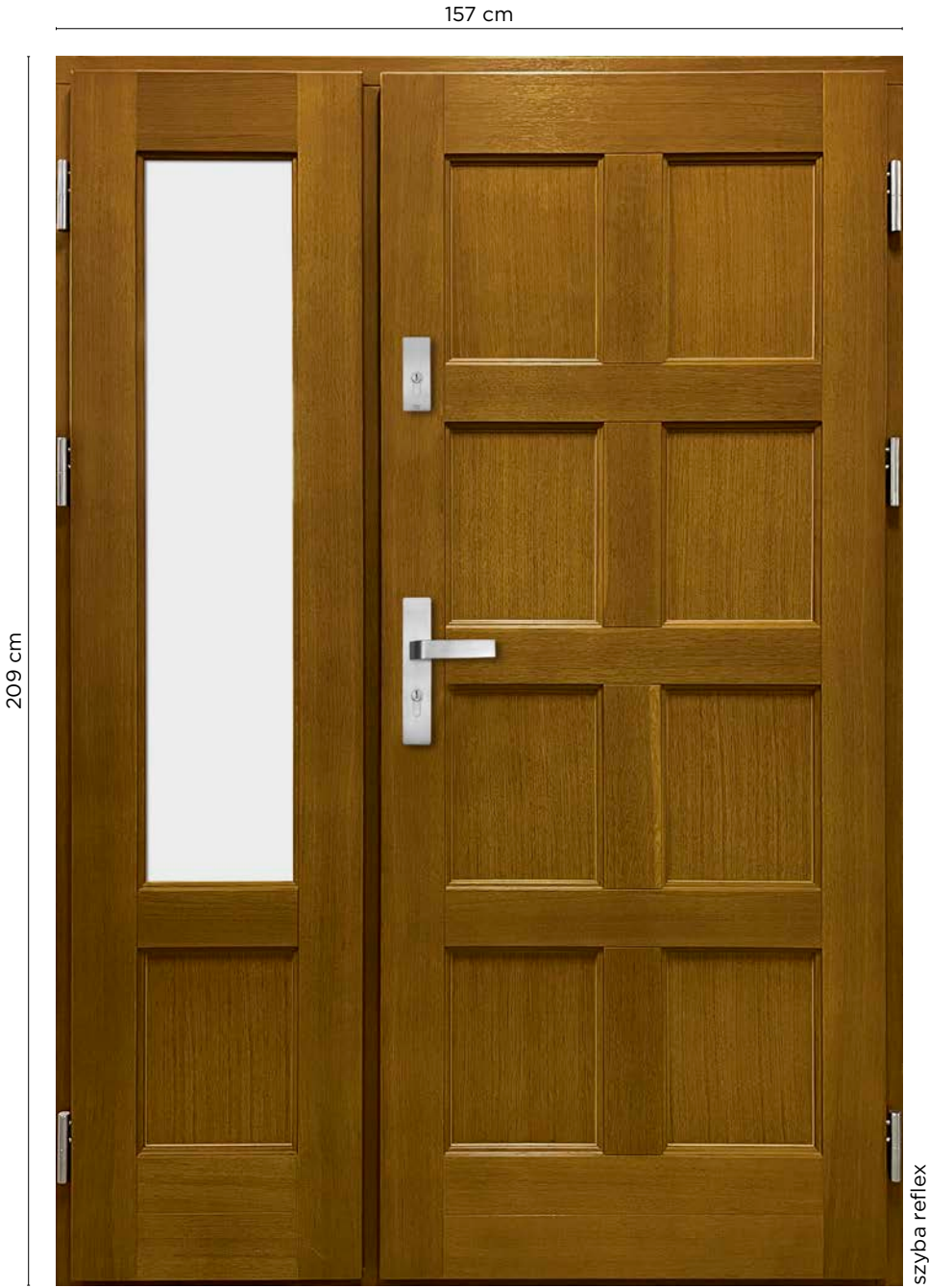
NS 45 Widok od zewnątrz Dostawka stała - imitacja skrzydła
