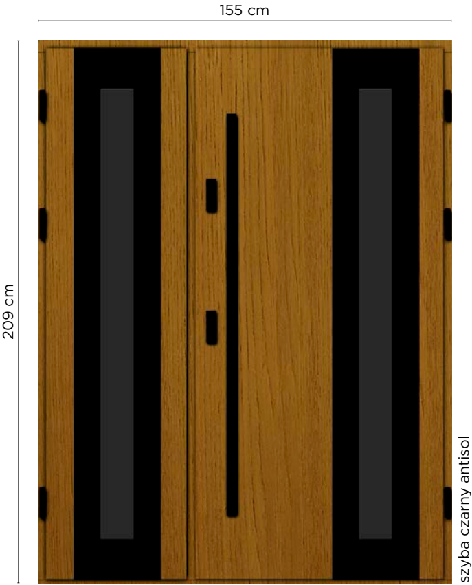
NS 38 Widok od zewnątrz Dostawka stała - imitacja skrzydła
